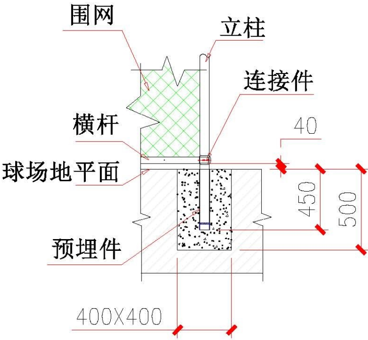
地面立柱基础图
